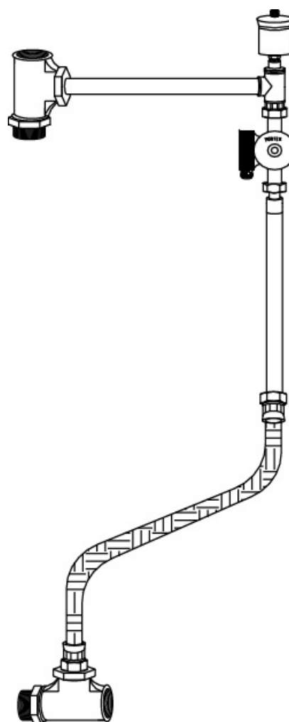
Schéma type kit assemblé
